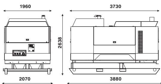
Монтируемый на раме
