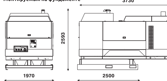
Монтируемый на фундаменте
