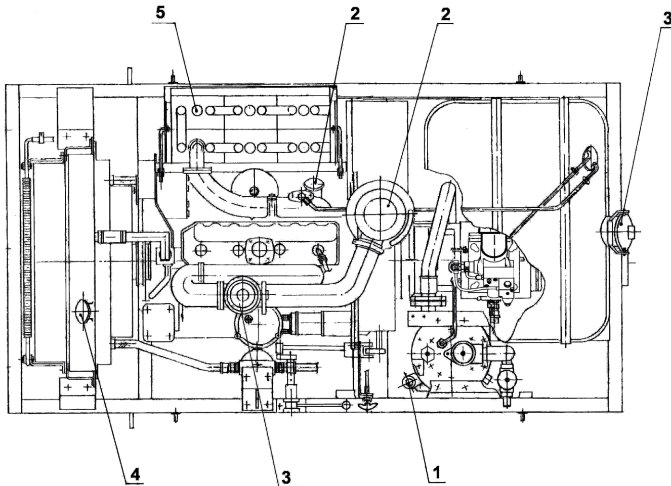
Рисунок В.15 - Схема заправки компрессорной станции ( см. приложение А )
