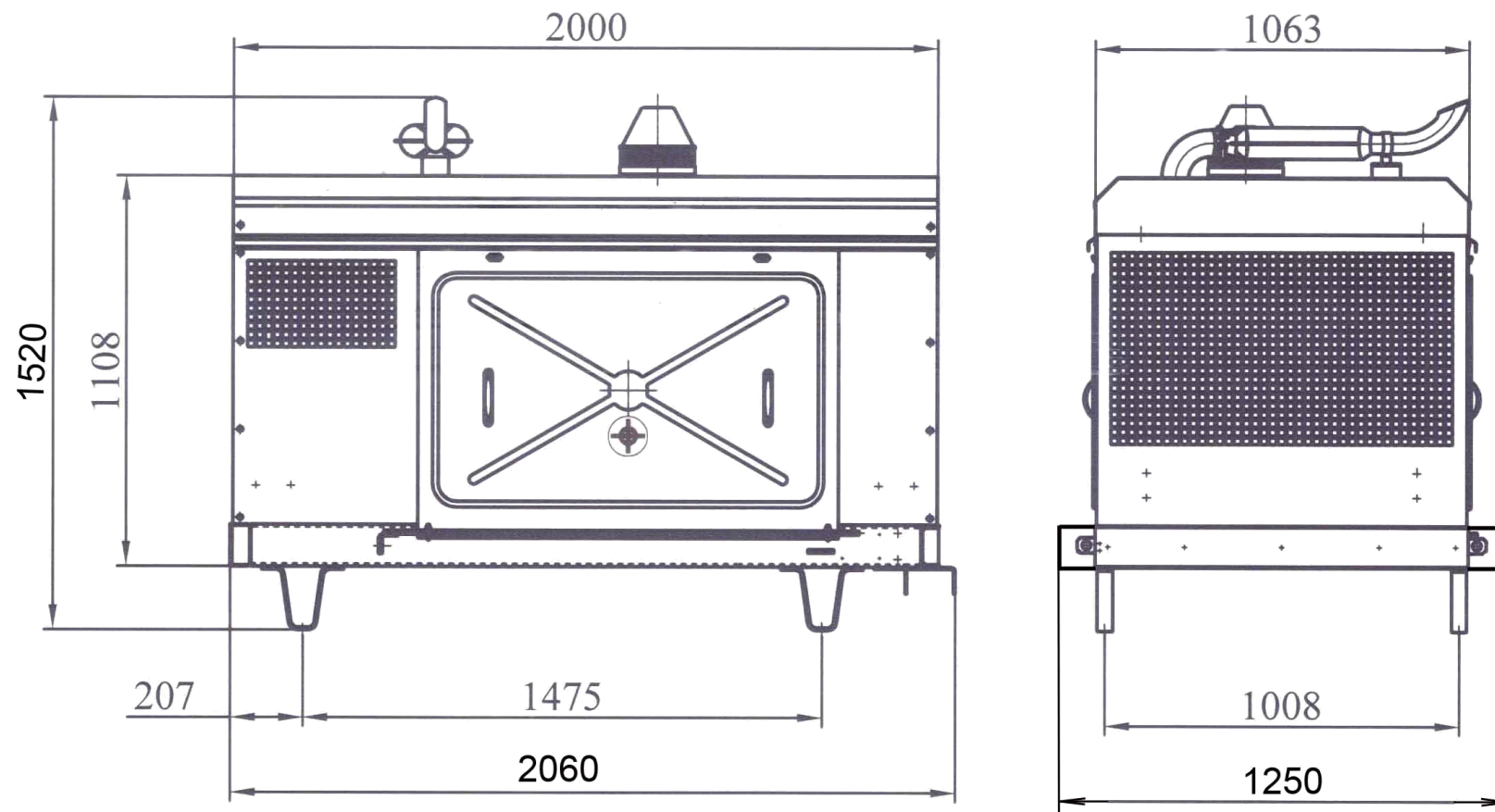
Рисунок В.1 - Габаритный чертеж компрессорных станций ЗИФ-ПВ5/1,0 (МЗА9-05). Исполнение на раме.
